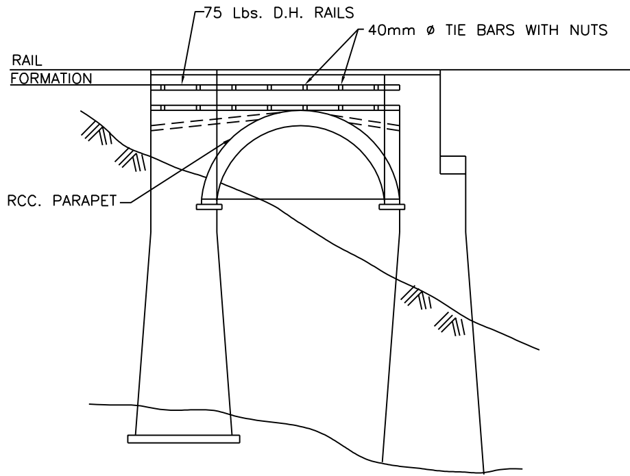
उद्विष्ट ELEVATION
