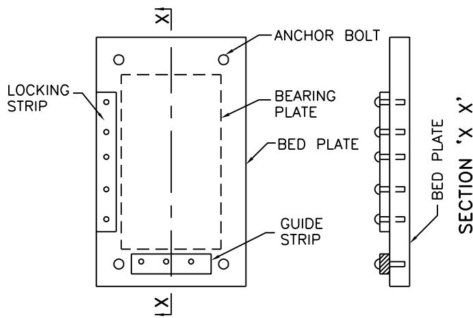
तलविज्ञेप PLAN
