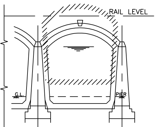
आंशिक काट उद्दिष्ट PART SECTIONAL ELEVATION
