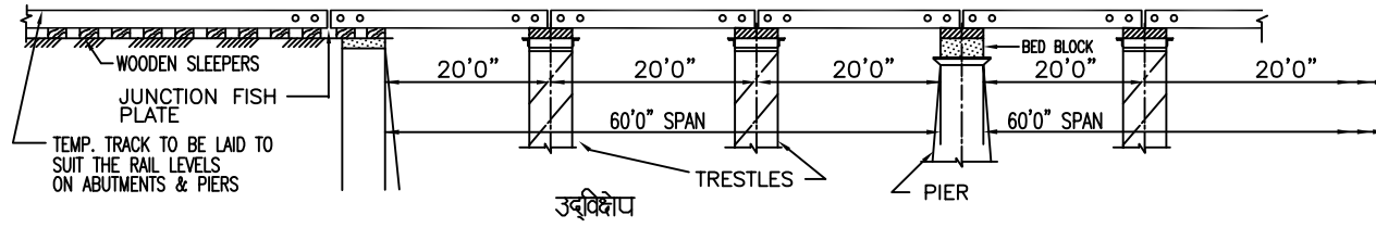
उदृष्टि ELEVATION
