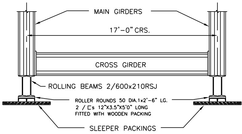
अनुप्रस्थ काट A-A CROSS SECTION A-A
