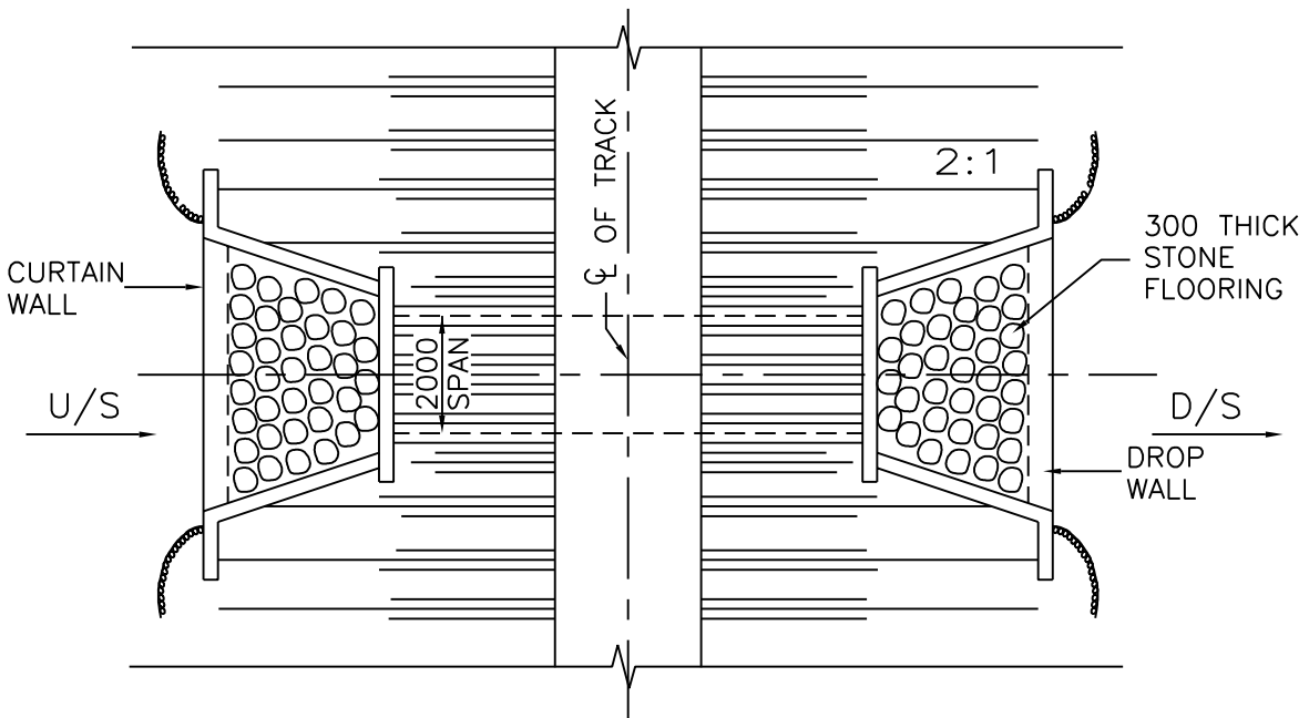
तलविक्षेप PLAN
