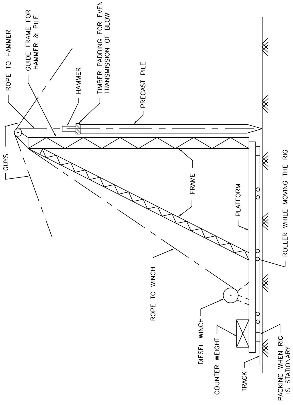
पूरे दृष्टा पाइलों को ठोकने के लिए प्रयुक्त रिग RIG USED FOR DRIVING PRE-CAST PILES
