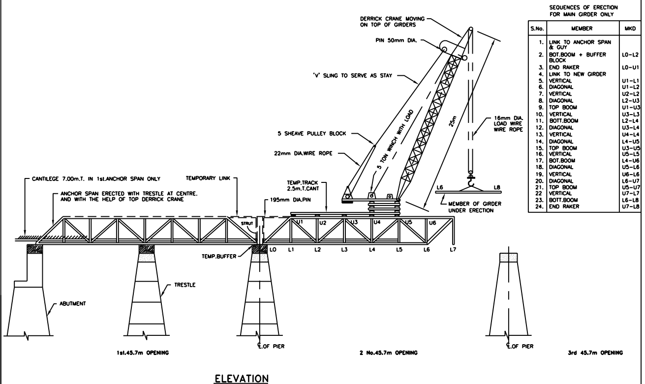
ELEVATION
