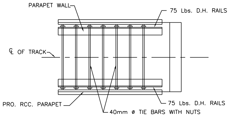
तलविष्ट PLAN
