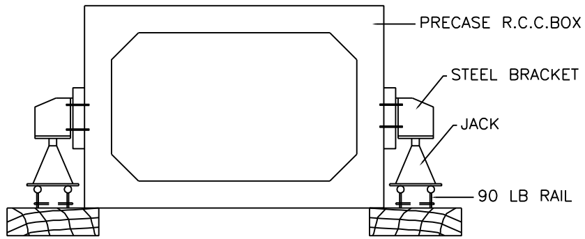
काट सी-सी SECTION 'C-C'
