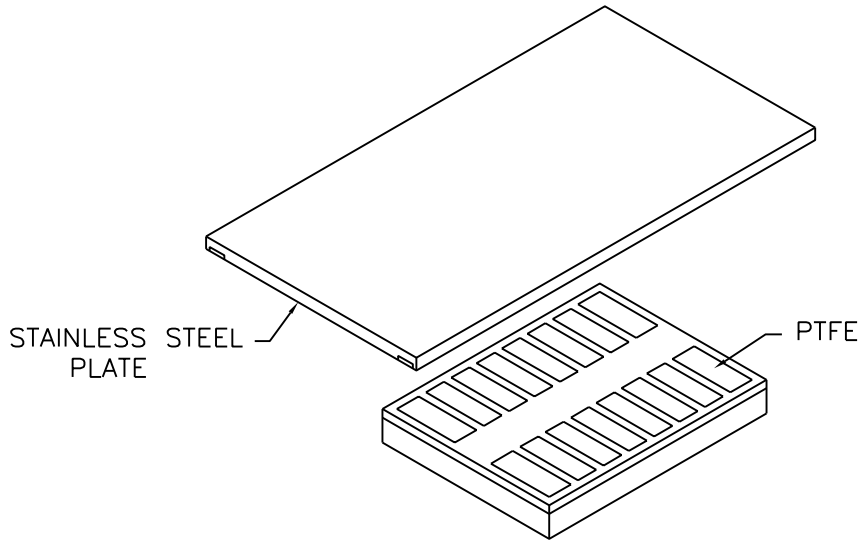
पी. टी. एफ. ई. बेयरिंग PTFE BEARING
