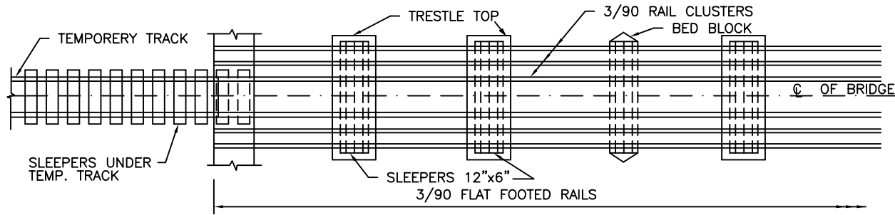
तलदृष्टि PLAN
