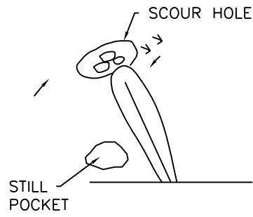
झुके हुए स्पर REPELLING SPUR
