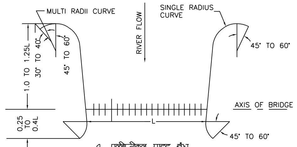
4. एल्लिप्टिकल गाइड बंध 4 ELLIPTICAL GUIDE BUND
