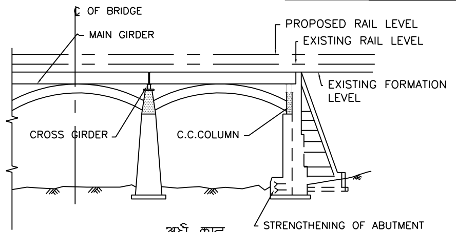
अर्ध काट HALF SECTION
