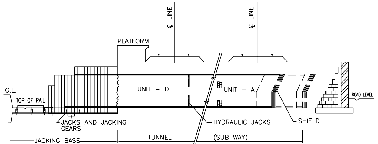
अनुप्रस्थ काट CROSS SECTION
